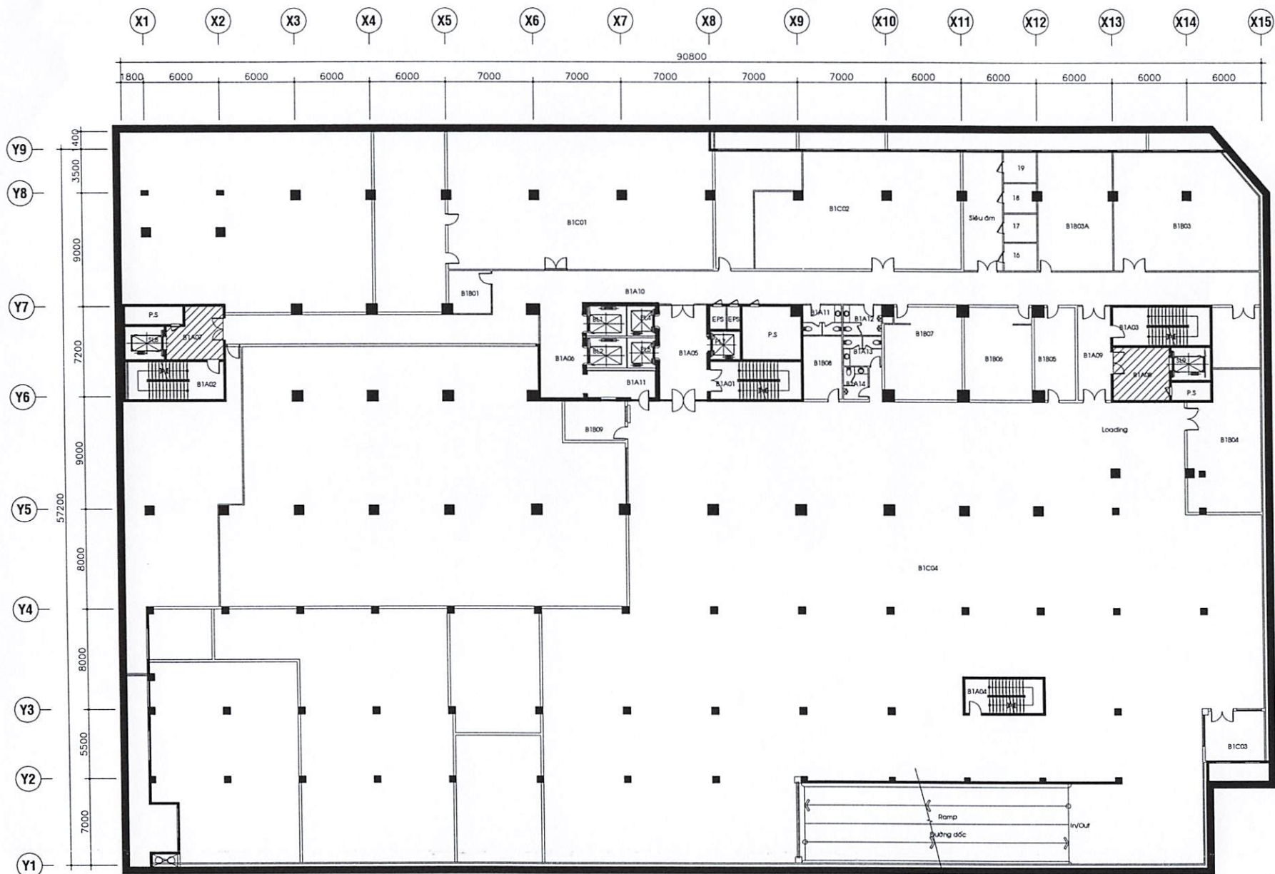
MẶT BẰNG TẦNG HẦM 1
