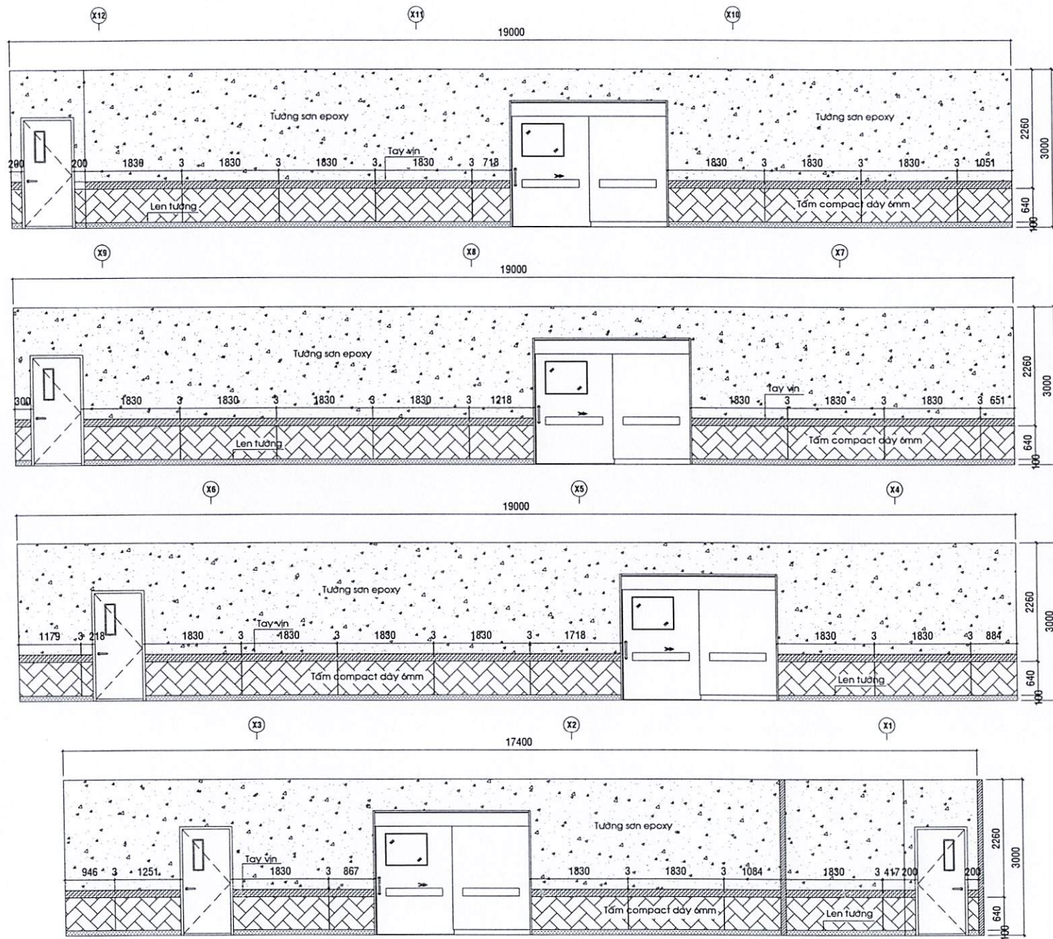
HƯỚNG NHÌN 2 LẦU 2
