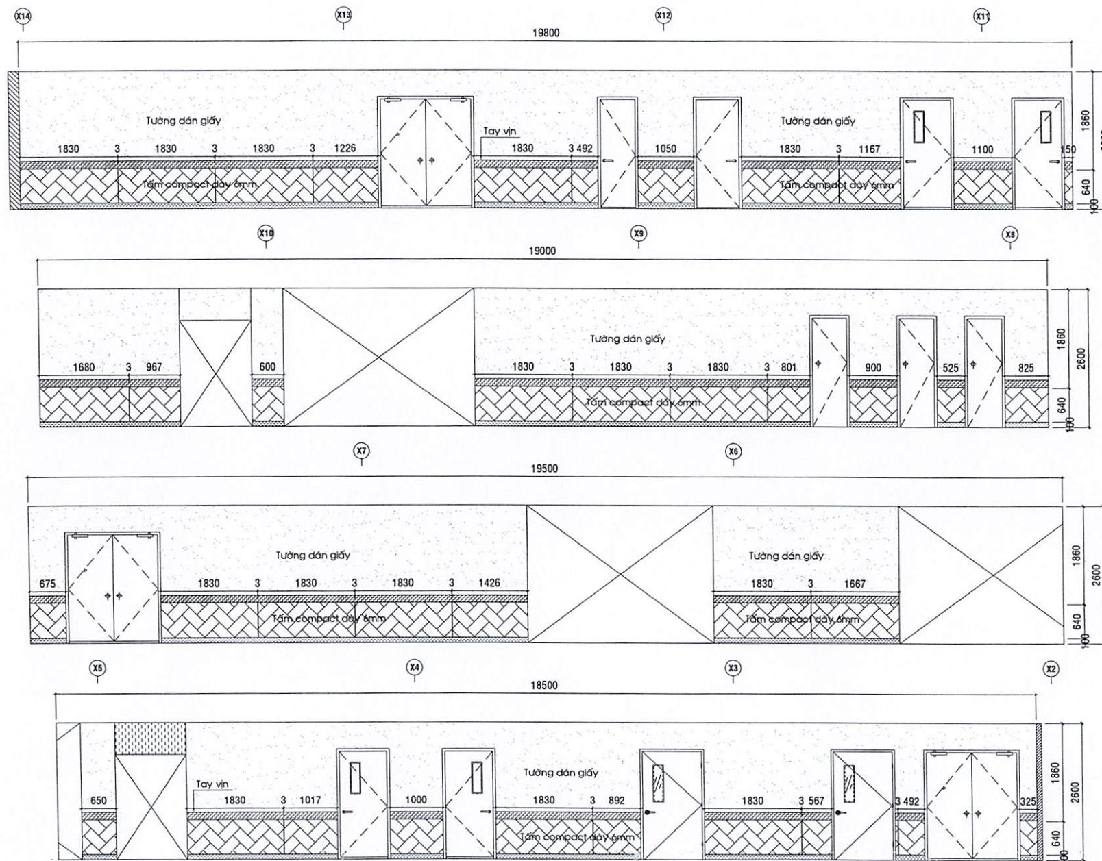
HƯỚNG NHÌN B LẦU 14
