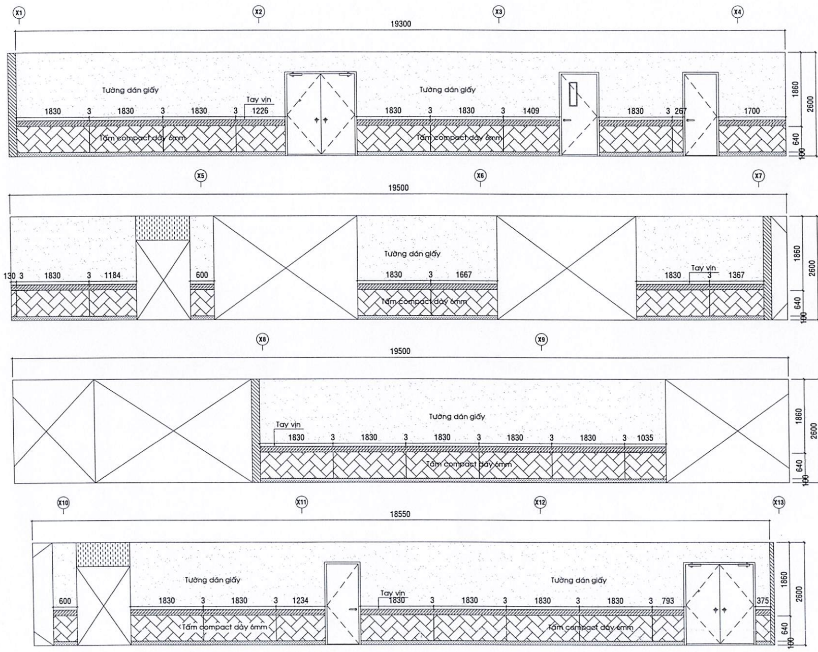
HƯỚNG NHÌN C LẦU 7
