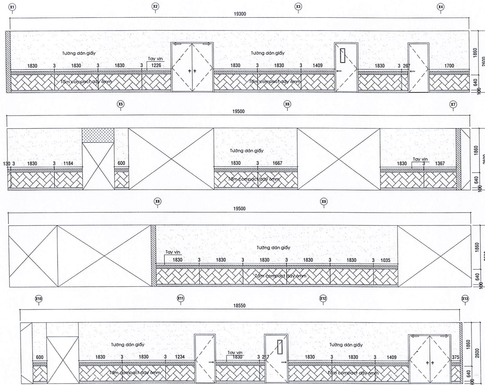
HƯỚNG NHÌN C LẦU 8 - 14
