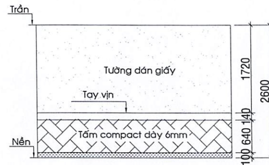
MẶT ĐỨNG ĐIỂN HÌNH LẦU 6
