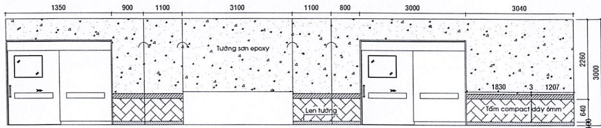
HƯỚNG NHÌN 9 LẦU 2
