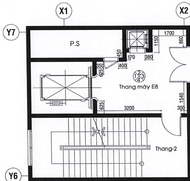
SẢNH THANG MÁY E8 (Lầu 2)
