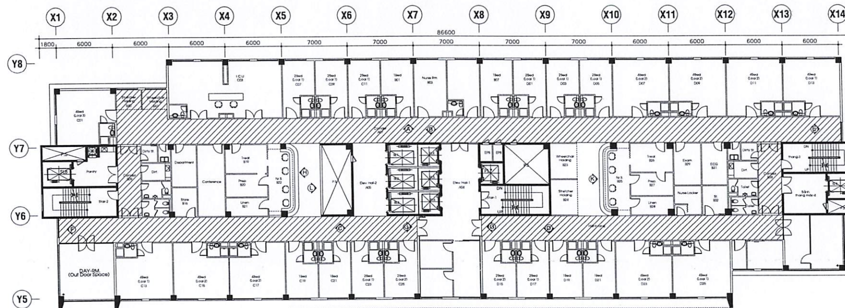
MẶT BẰNG LẦU 7
