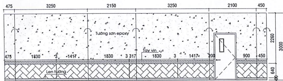
HƯỚNG NHÌN 3 LẦU 2
