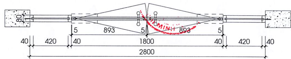
MẶT CẮT 1-1 (Tỷ lệ 1/30)
