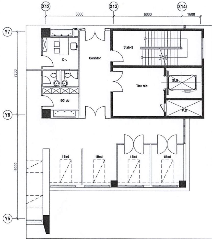
MẶT BẰNG LẦU 5 TRƯỚC KHI SỬA CHỮA
