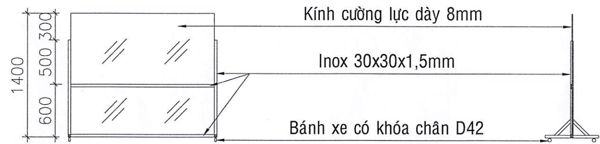
MẶT ĐỨNG VÁCH KÍNH VK2
