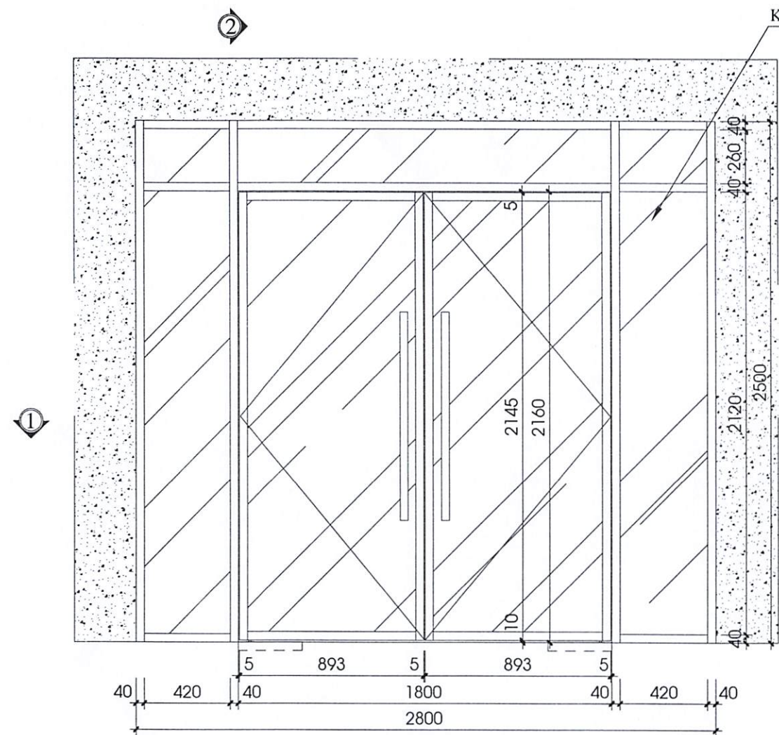
MẶT ĐỨNG VÁCH KÍNH VK3 (Tỷ lệ 1/30)
