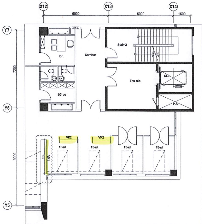
MẶT BẰNG LẦU 5 SAU KHI SỬA CHỮA
