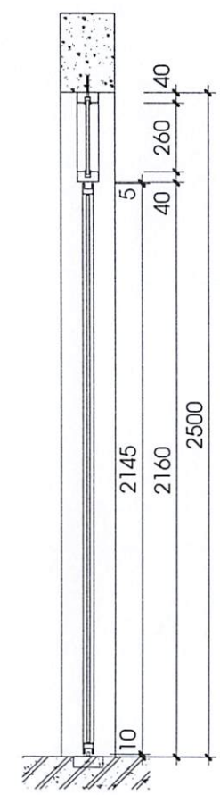
MẶT CẮT 2-2 (Tỷ lệ 1/30)
