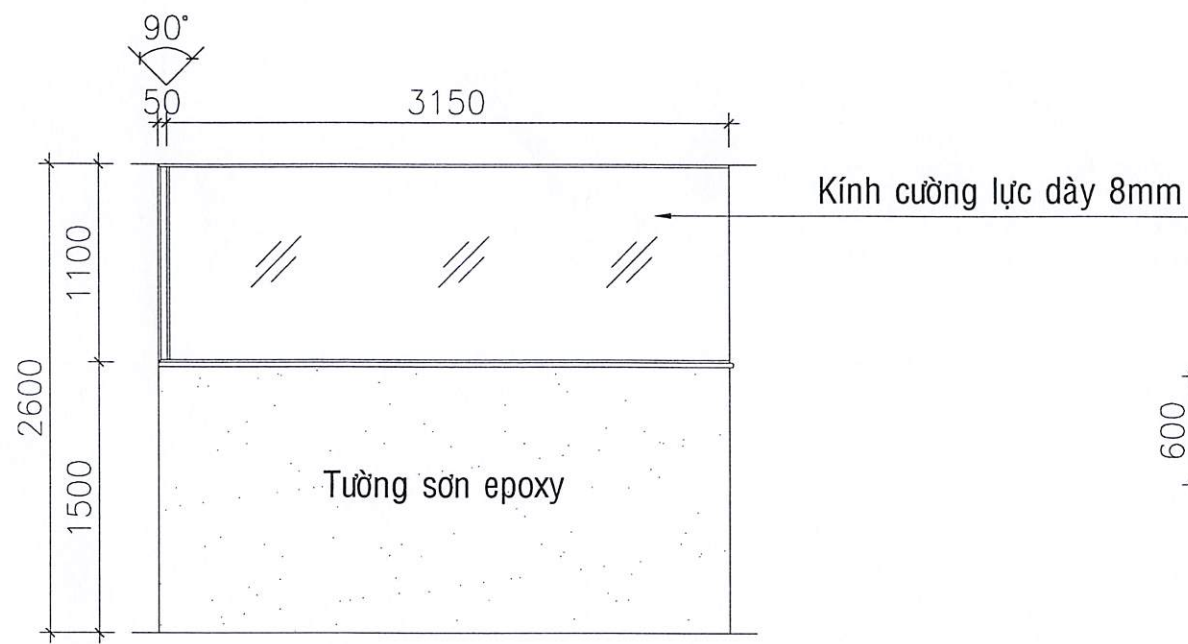
MẶT ĐỨNG VÁCH KÍNH VK1
