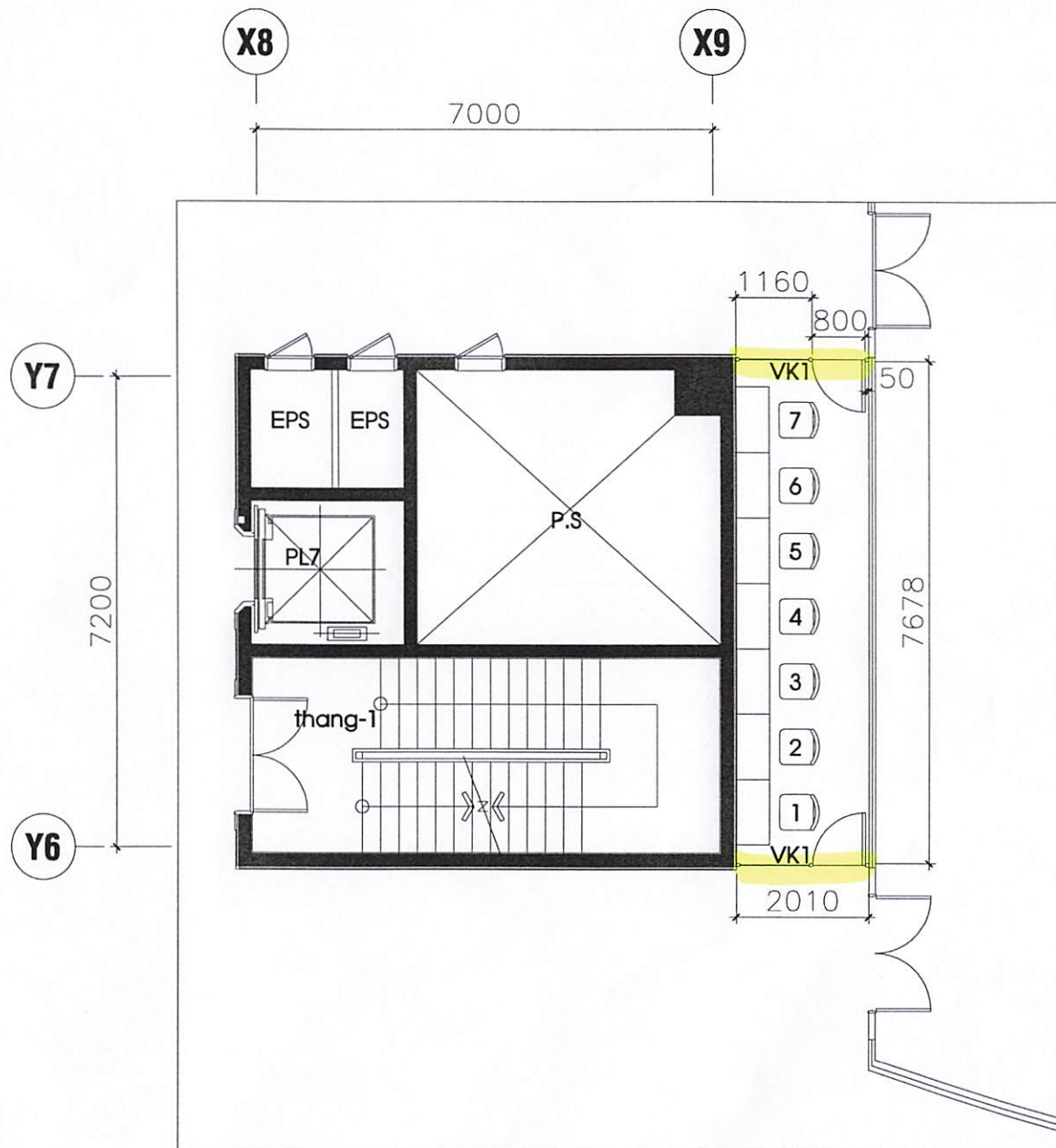
MẶT BẰNG LẦU 3 SAU KHI SỬA CHỮA
