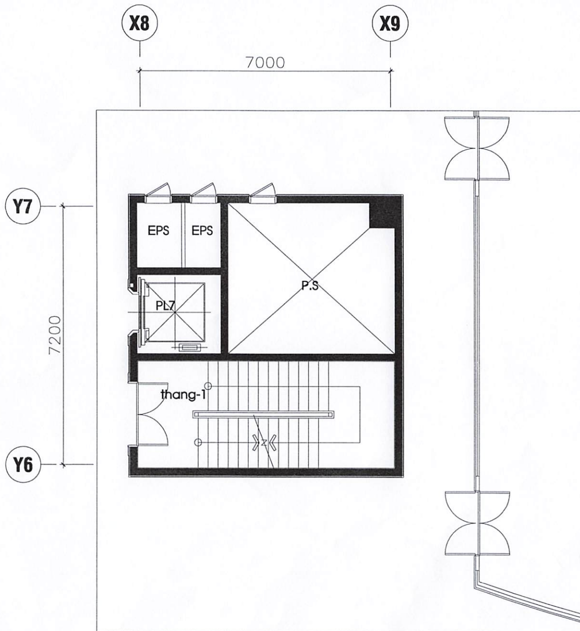
MẶT BẰNG HIỆN TRẠNG LẦU 3
