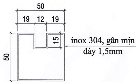
CHI TIẾT D2
