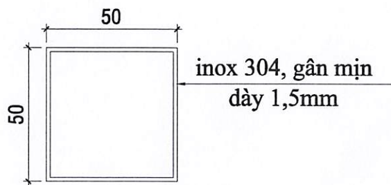
CHI TIẾT D1
