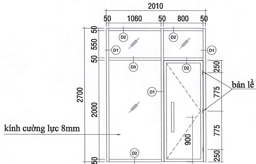
VÁCH KÍNH VK1
